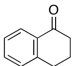
\alpha -tetralone
